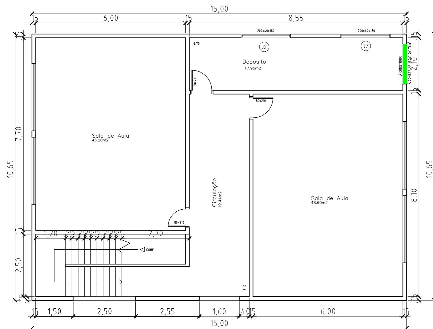
6 PLANTA BAIXA 2º PAVTO. ESC 1/75
